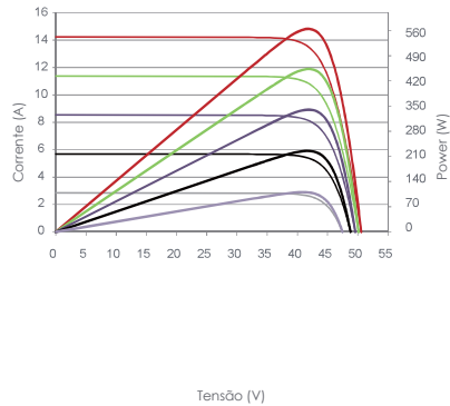
Curvas de corrente-tensão e potência-voltagem (565W)
