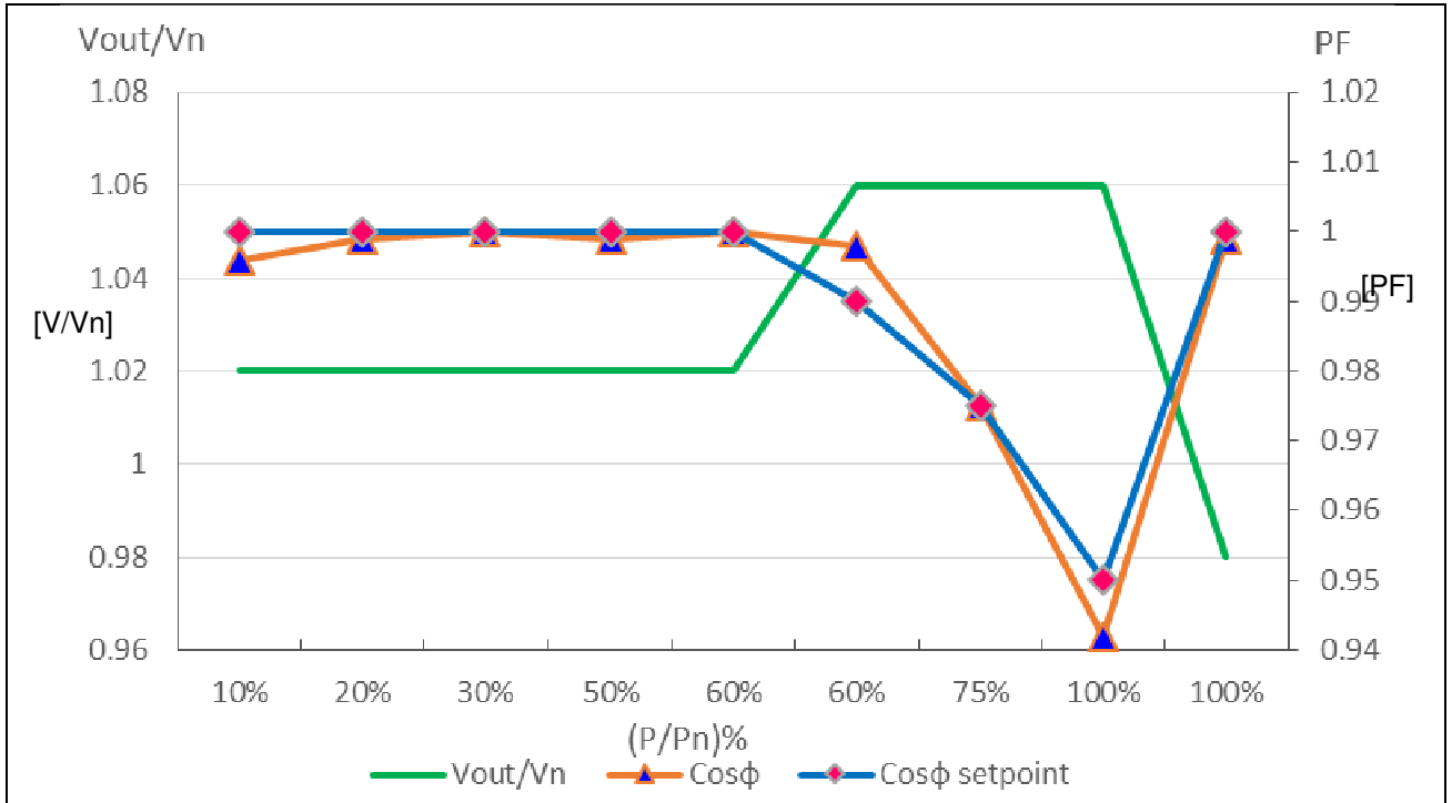
Gráfico produção de potência reativa de acordo com uma característica Curva do Fator de Potência Graph reactive power production according to a characteristic Power Factor Curve
