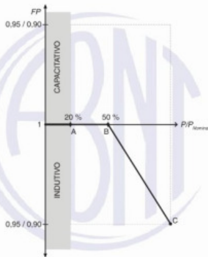
Gráfico produção de potência reativa de acordo com uma característica Curva do Fator de Potência Graph reactive power production according to a characteristic Power Factor Curve
